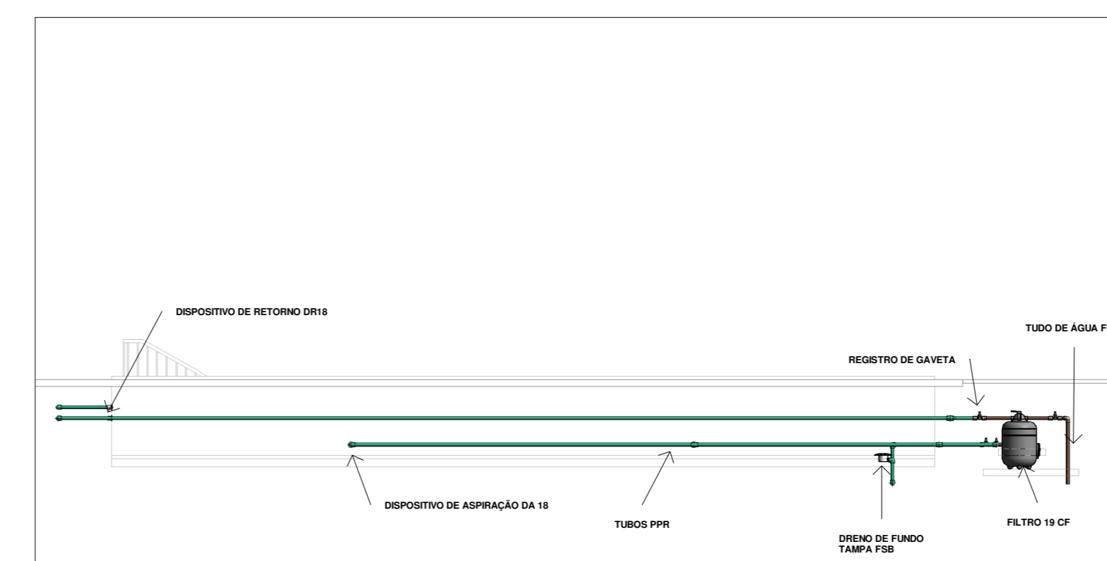
Corte 4 ESCALA: 1 : 100
