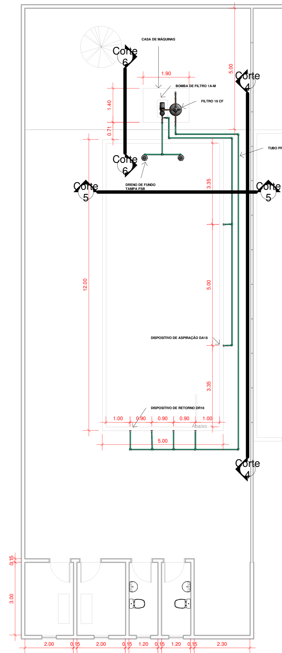
HIDRAULICO ESCALA: 1 : 100
