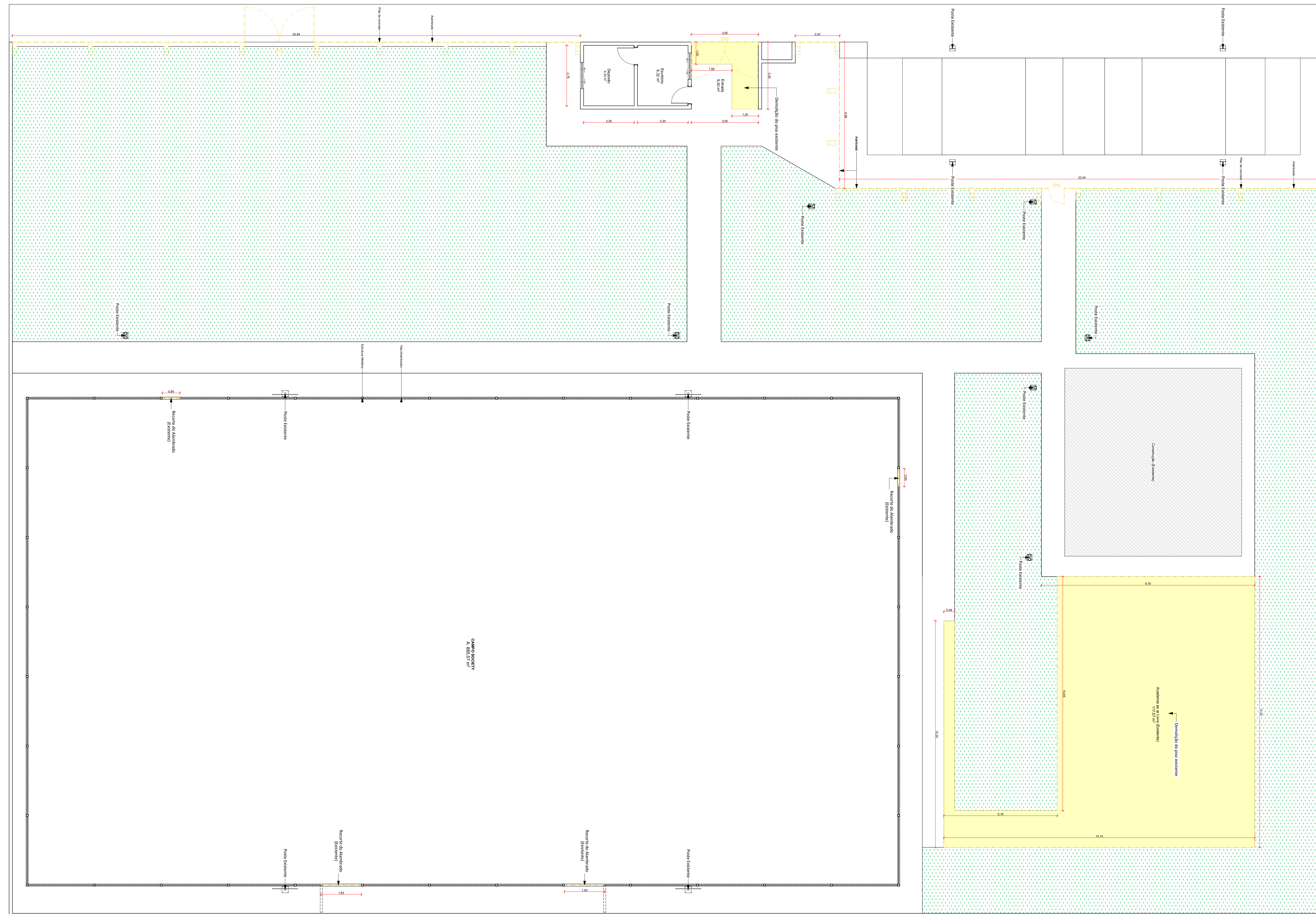
PROJETO DE DEMOLIÇÃO Escala: 1:75
