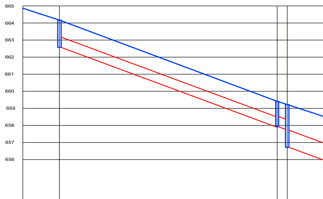
CORTE CC-DETALHE EM PERFIL DA REDE DRENAGEM SEM ESCALA
