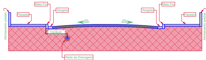
CORTE CC-DETALHE EM PERFIL DA REDE DRENAGEM SEM ESCALA
